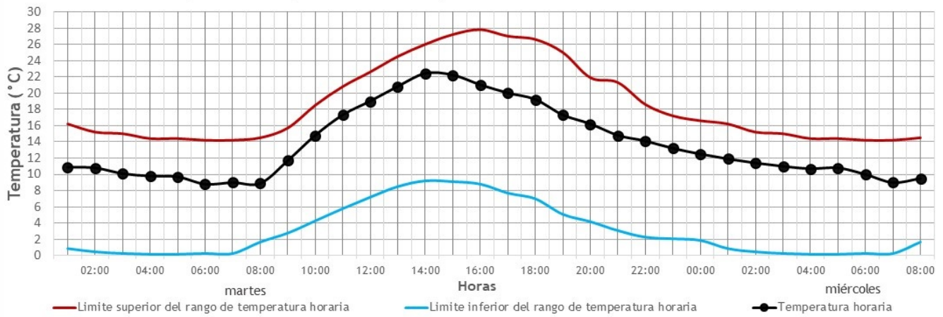
Temperatura horaria para los días martes 12 y miércoles 13 de enero de 2021
