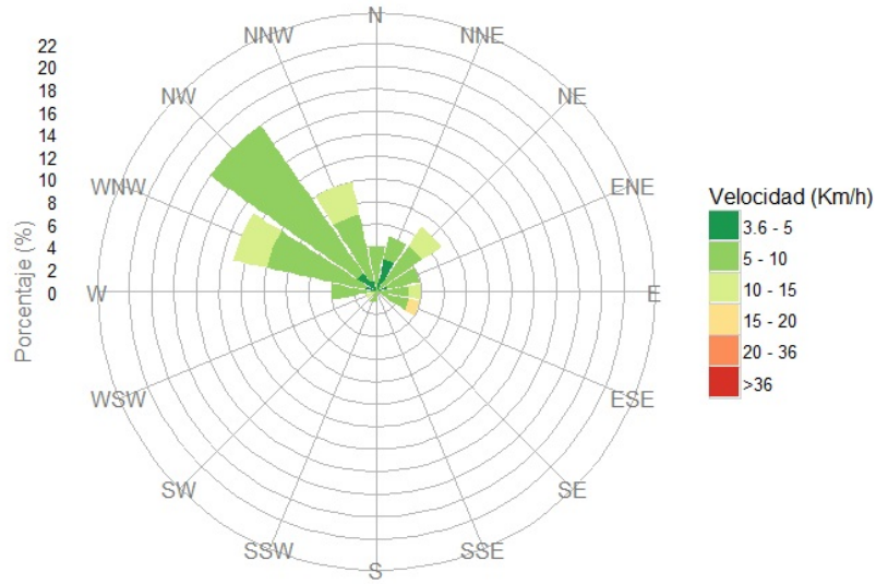
Rosa de los vientos Observatorio Meteorológico Central del día lunes 21 de octubre de 2019 Datos cada 15 min.
