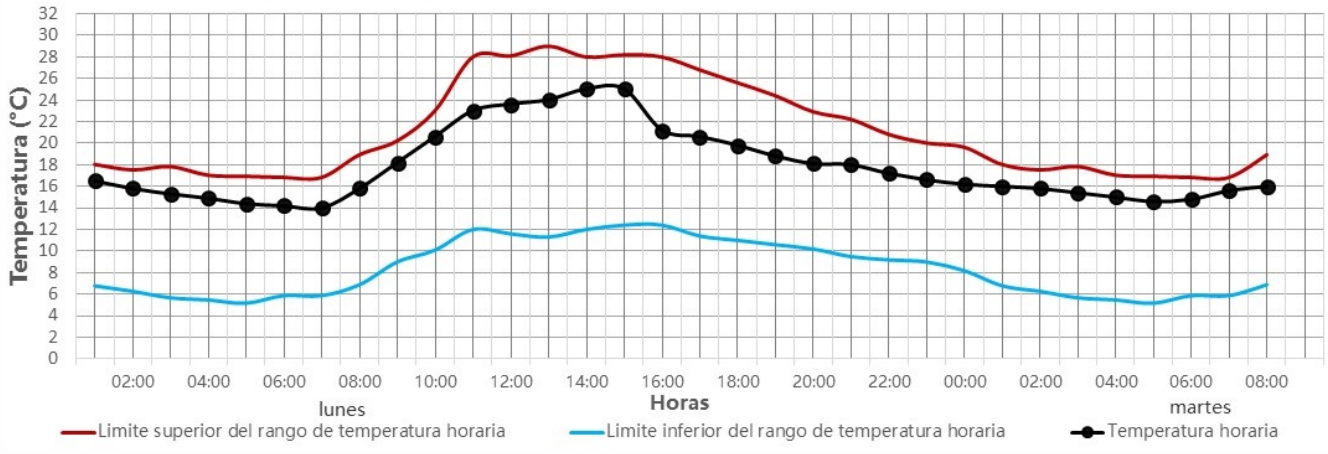
Temperatura horaria para los días lunes 21 y martes 22 de octubre de 2019
