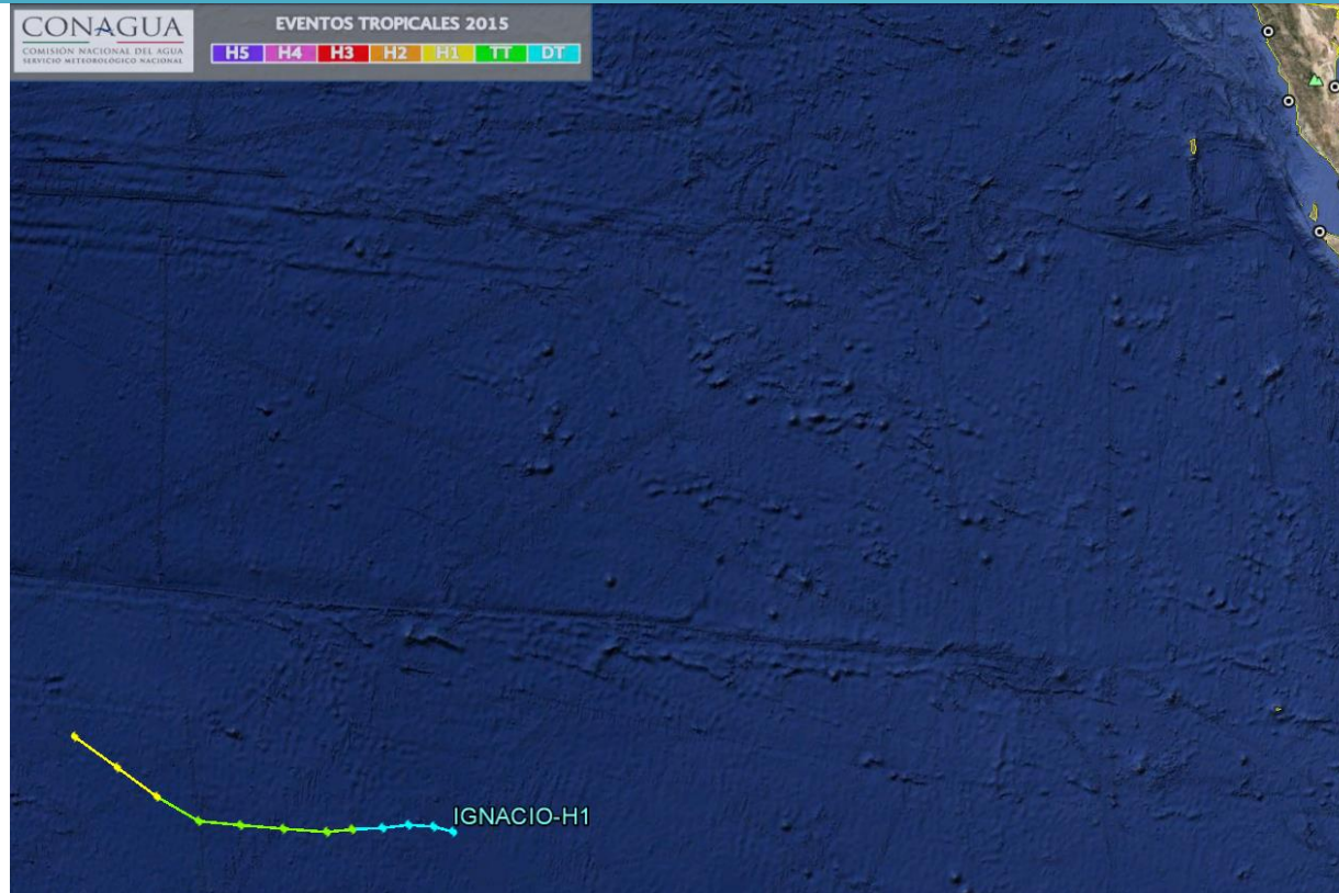
Trayectoria final del Huracán "Ignacio" del Océano Pacífico
