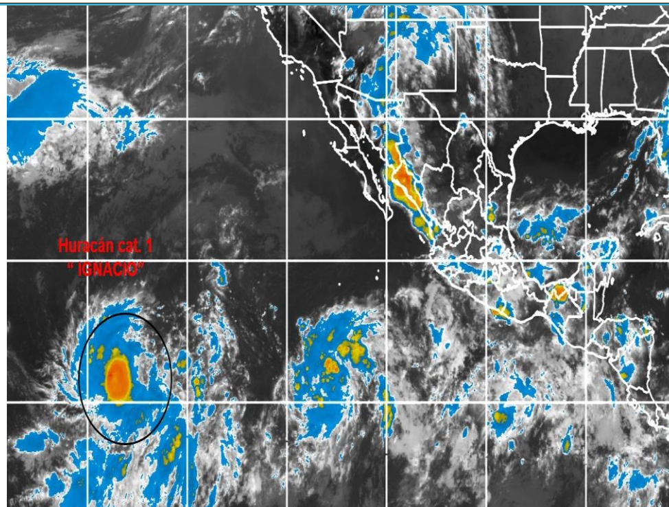
Imagen de satélite en canal Infrarrojo del Huracán "Ignacio" del Océano Pacífico.
