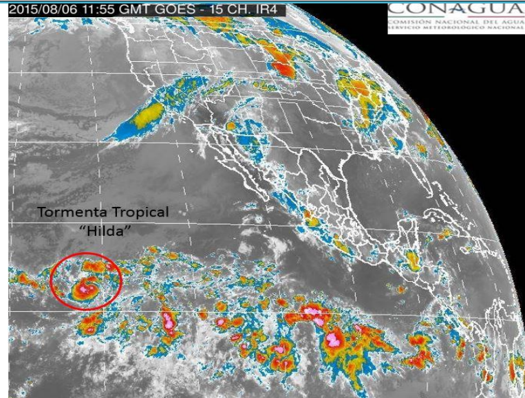
Imagen de satélite en canal infrarrojo de la tormenta tropical "Hilda" del Océano Pacífico.
