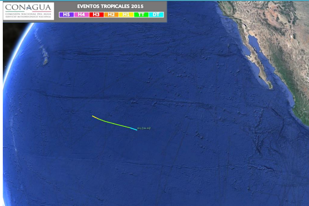
Trayectoria final del huracán "Hilda" del Océano Pacífico Nororiental
