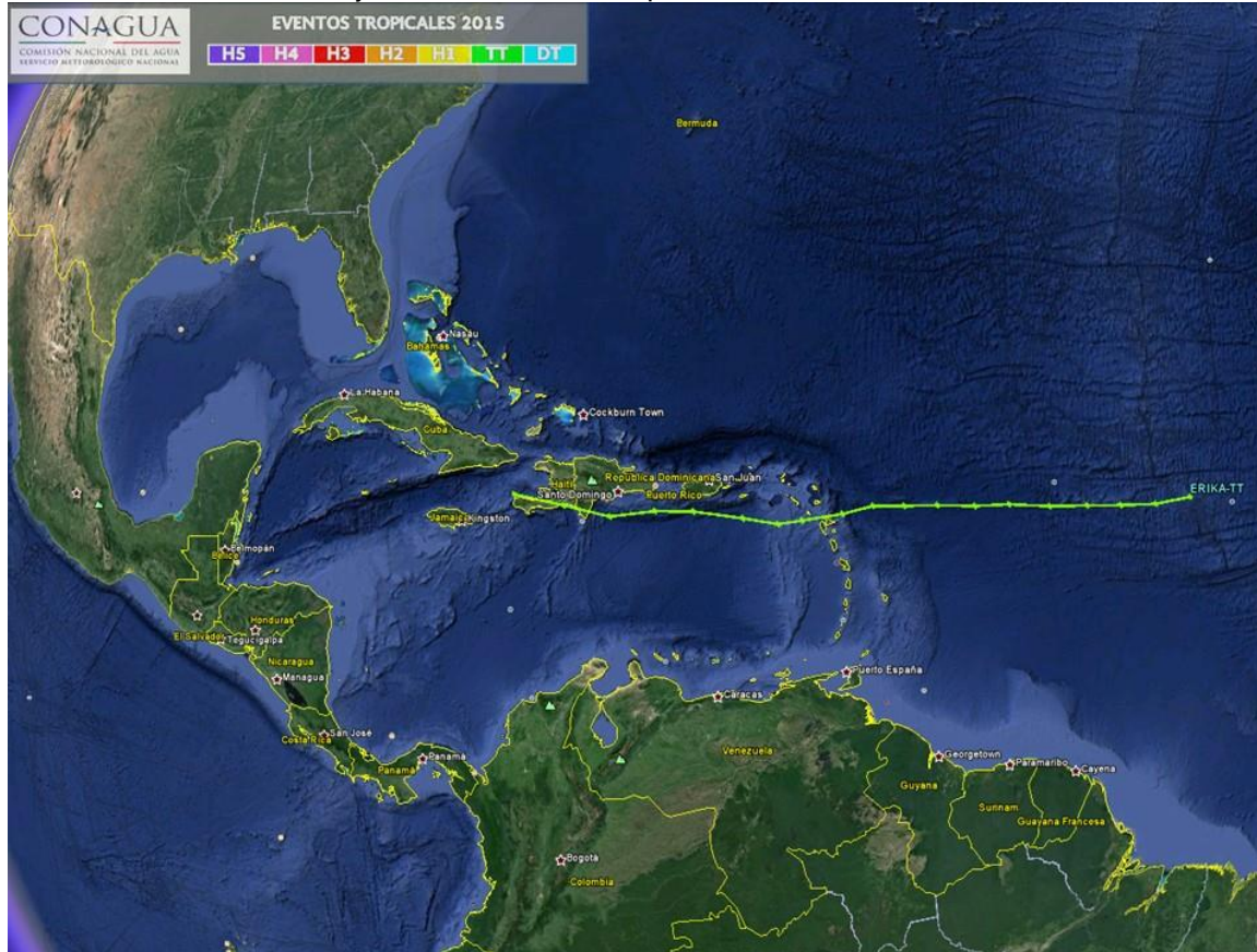
Trayectoria final de la Tormenta Tropical "Erika" del Océano Atlántico
