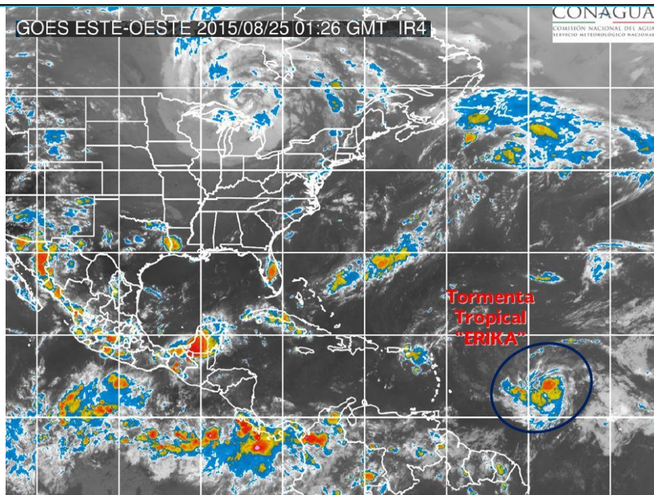
Imagen de satélite canal infrarrojo con la tormenta tropical "Erika" del Océano Atlántico. CNA-CGSMN - GOES-13 IR Agosto 24 a las 20:26 horas
